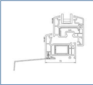
70 mm karm Illustreret som opluk med påmonteret alu-sålbænk
