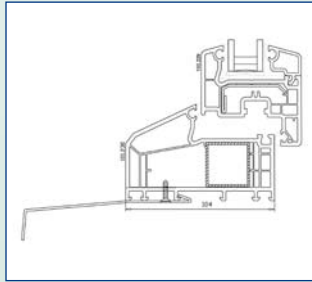
104 mm karm Illustreret som opluk med påmonteret alu-sålbænk
